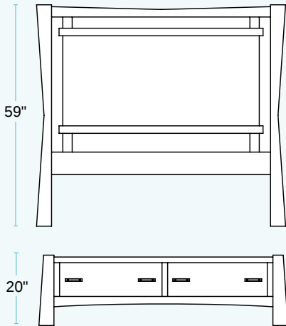
Bed with Footboard Drawer Unit • #62104 King . . . . . 83W • #62109 California King . . . . . 79W • #62105 Queen . . . . . 67W • #62106 Full . . . . . 61W • #62107 Twin . . . . . 45W
